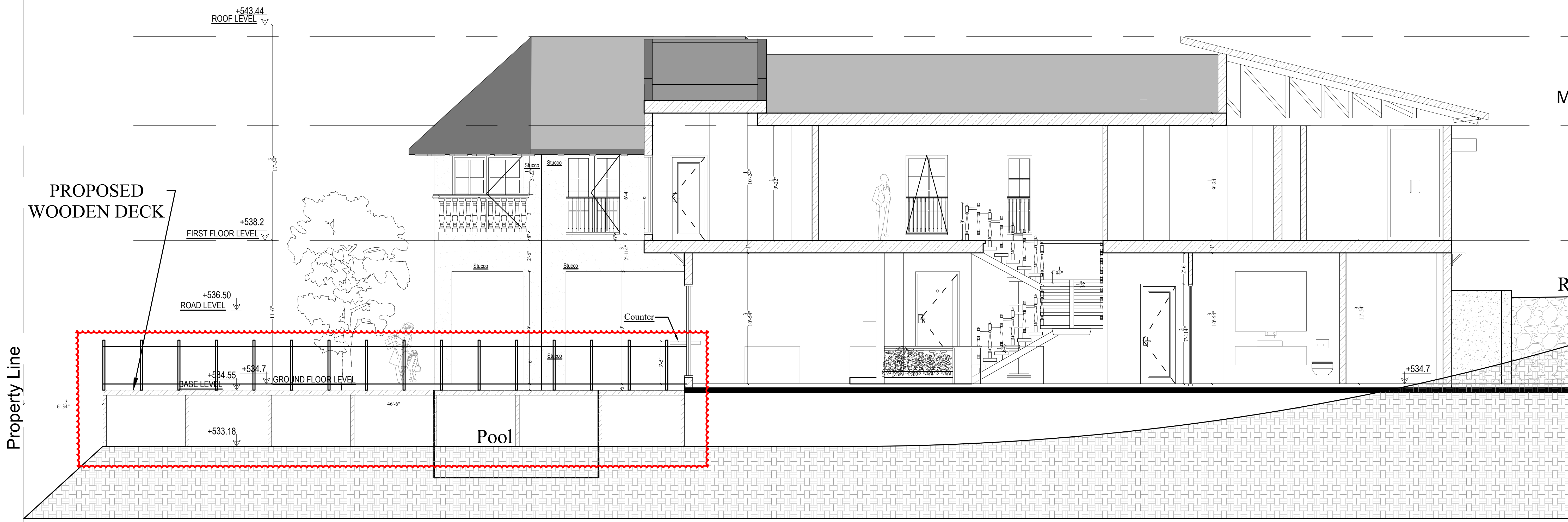
Section A-A Scale: 1/4"=1'
